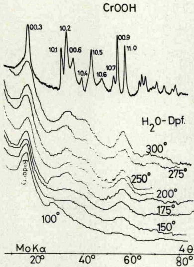
Fig. 7. Siehe Fig. 6, jedoch Wasserdampf-Atmosphäre. Zuerst ist das Diagramm von trigonal-rhomboedrischem CrOOH mitdensitometriert, zur Illustration der Fragwürdigkeit solcher Nachweise bestimmter Kristallarten.
